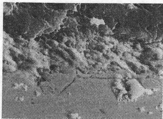
Mag. 400 X.
